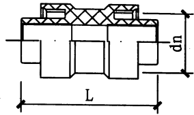
等径套管
