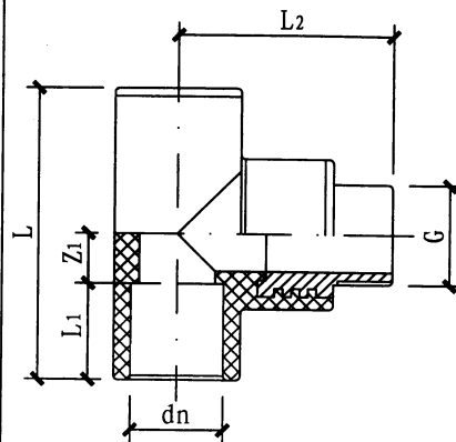
外螺纹三通
