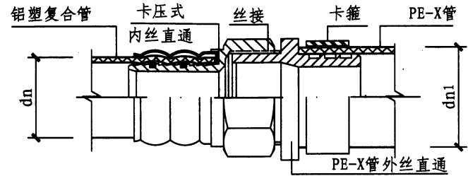
螺纹连接 (四)
