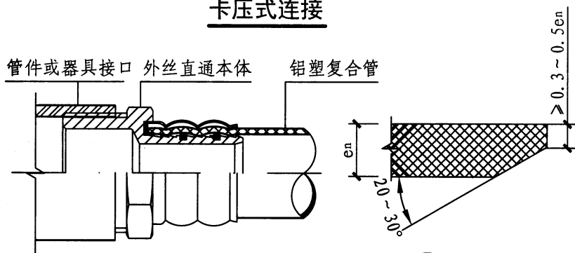
外丝直通连接
