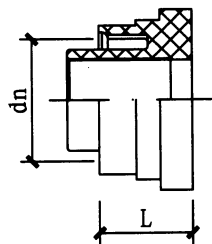
活接头熔件
