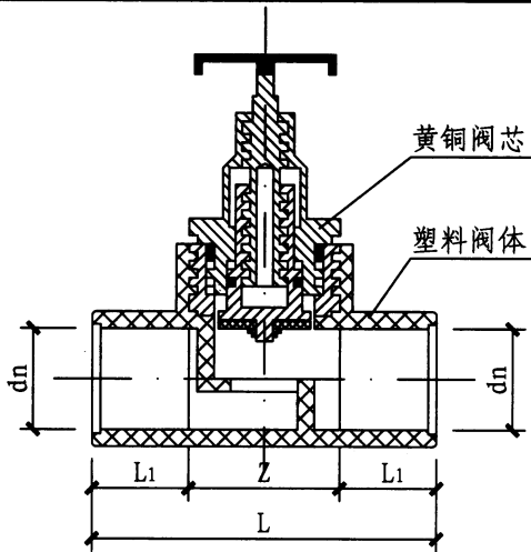
铜塑截止阀
