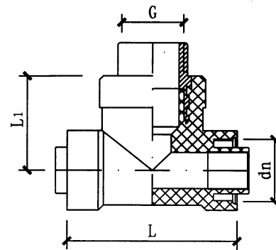
外螺三通
