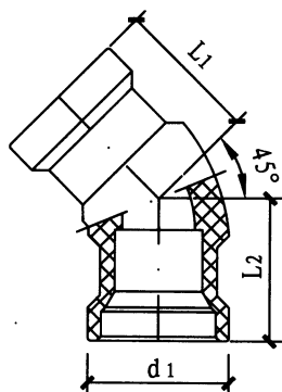
45° 弯头
