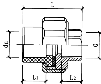
内螺纹活接头
