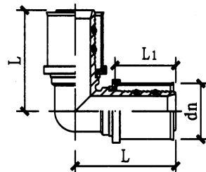
卡压式等径弯头
