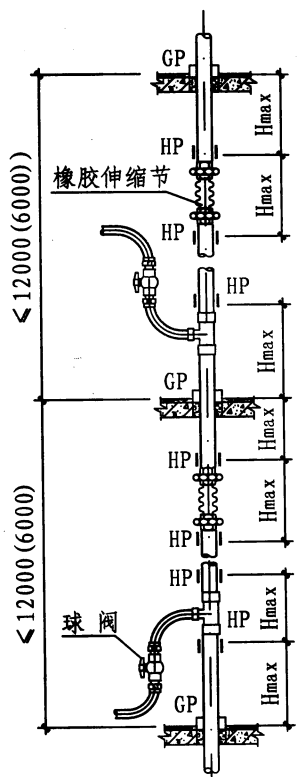
层高 ≤ 12.0 (6.0) m (dn ≤ 32)
