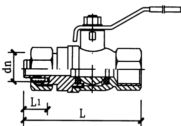
卡套式球阀
