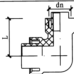
90°弯头
