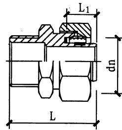
卡套式外丝直通
