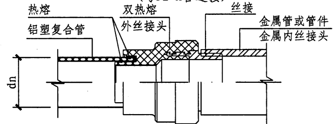
螺纹连接 (五)
